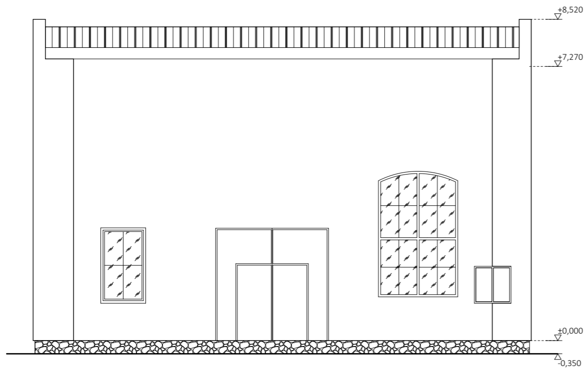
POHLED PB03
