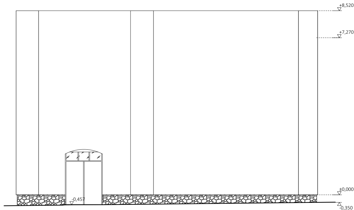
POHLED PB02
