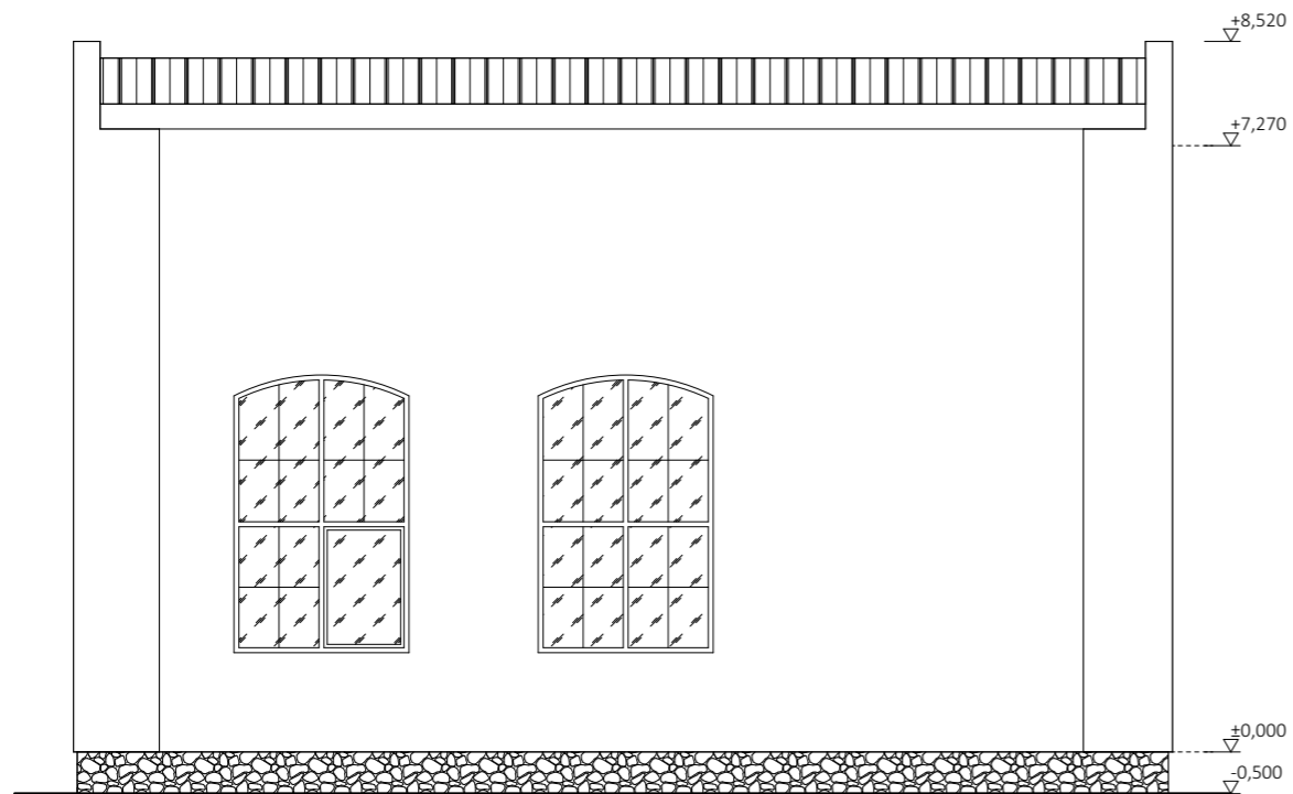
POHLED PB01
