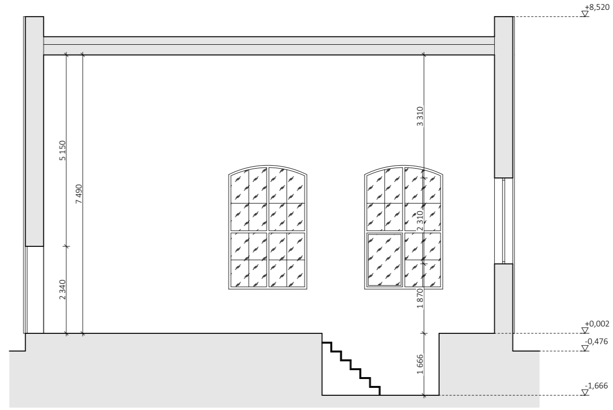
ŘEZ B02
