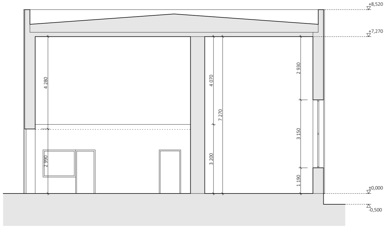
ŘEZ B01
